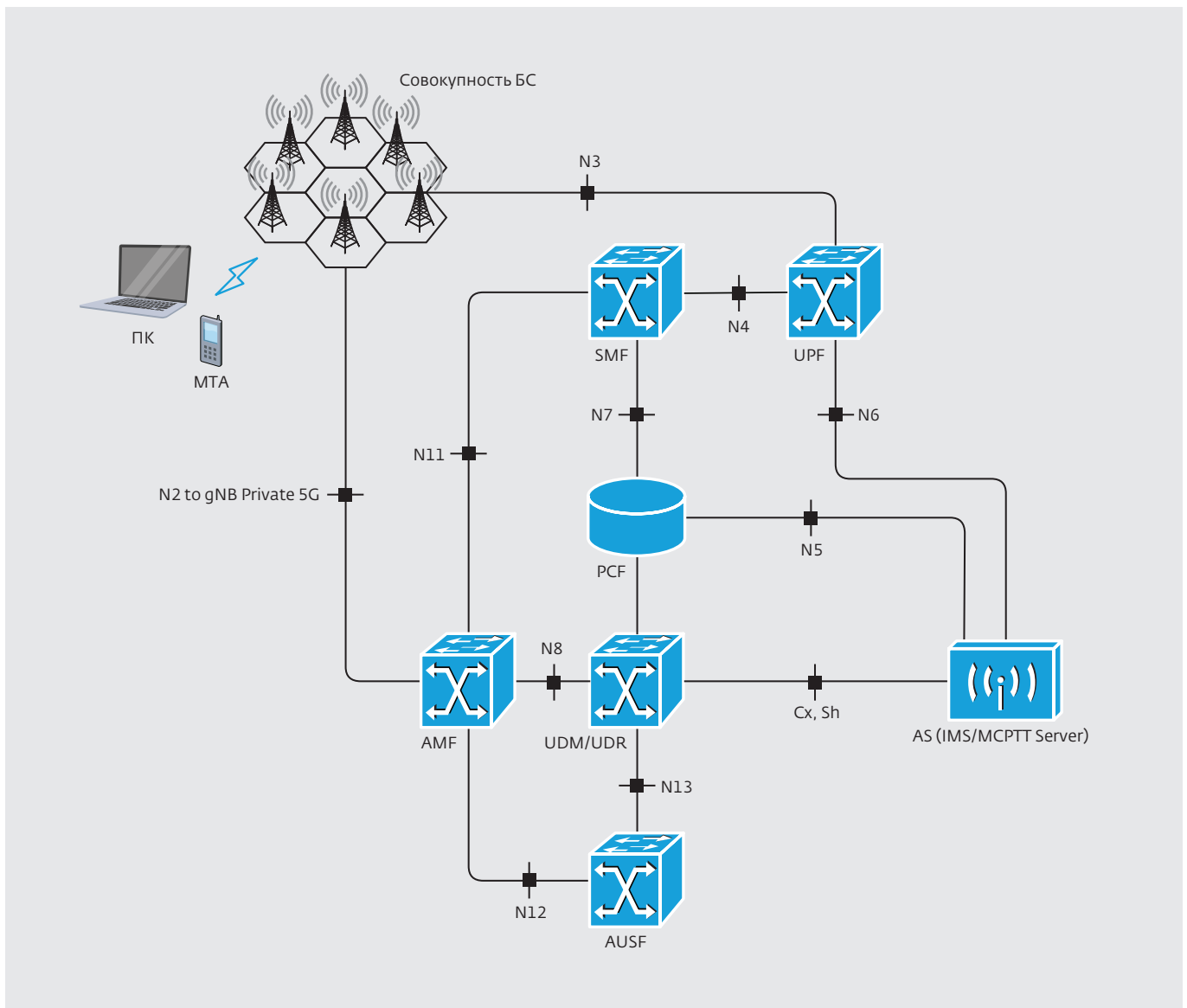
Рис.5. Архитектура системы для реализации услуг VoNR/MCPTT
