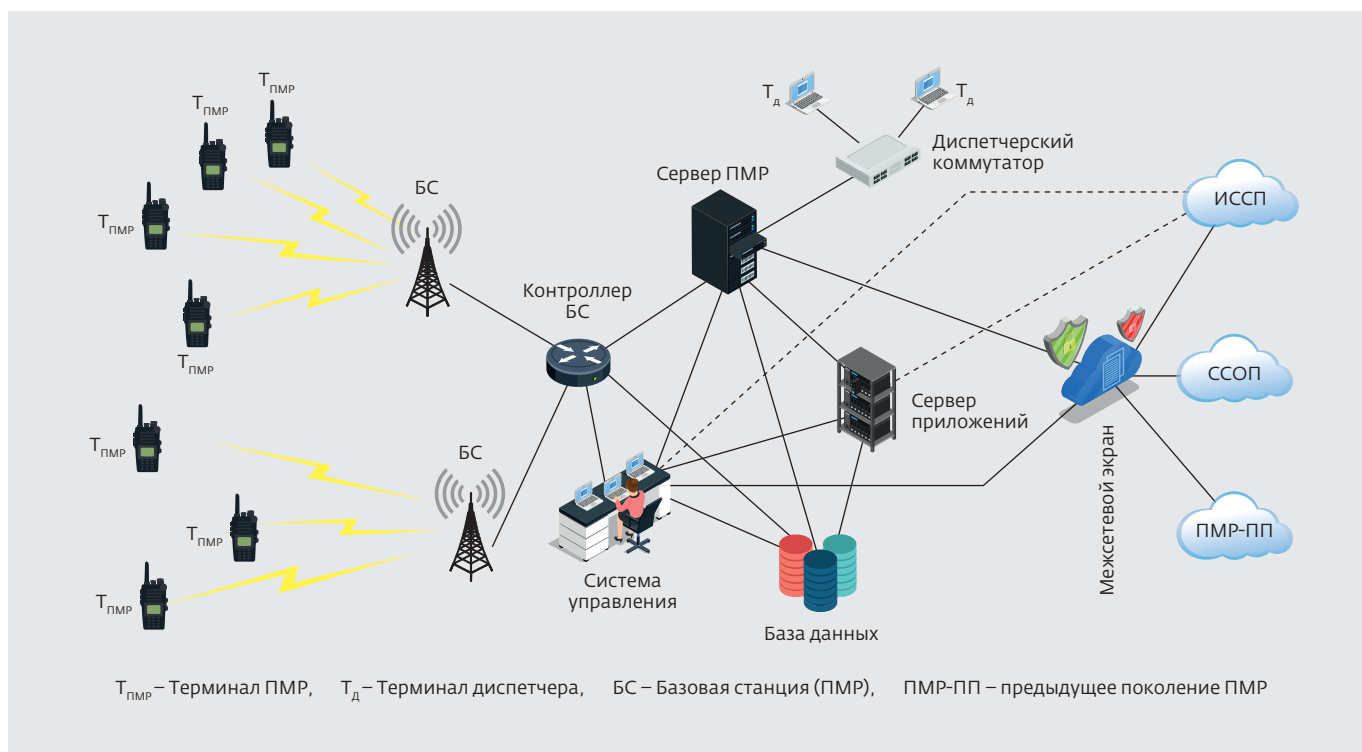
Рис.1. Функциональная модель перспективной системы ПМР
