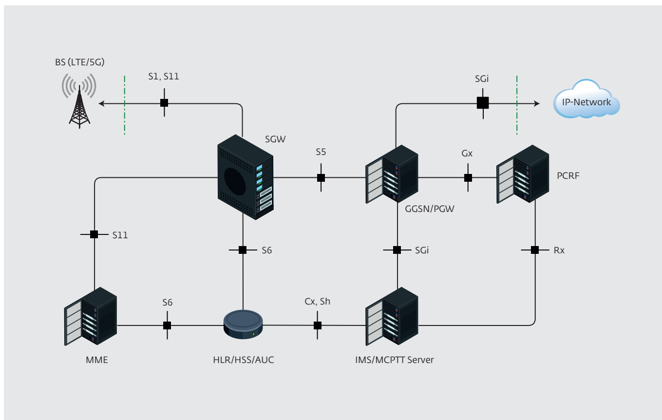
Рис.4. Структура ядра системы Private LTE
