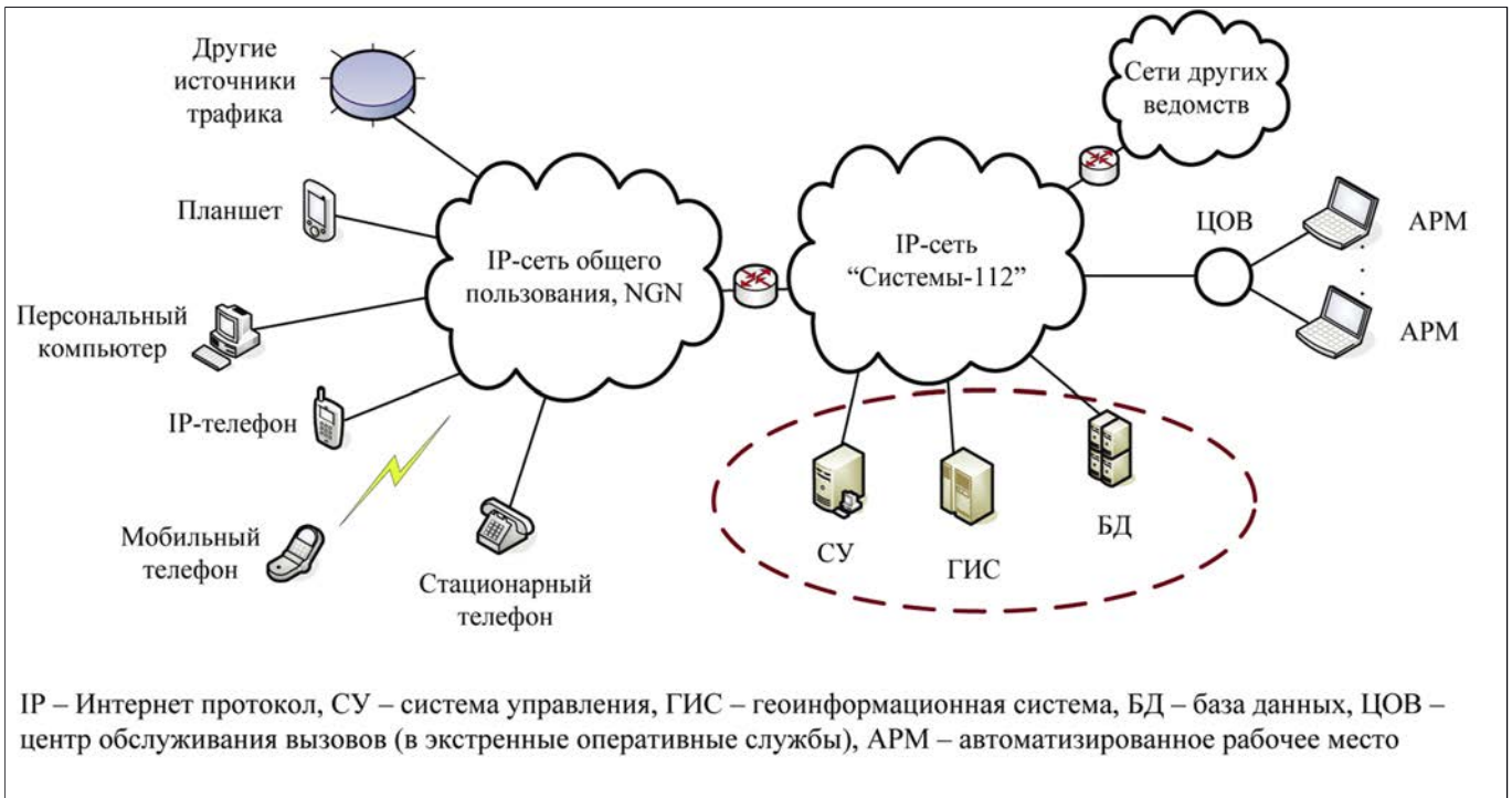
Рис. 2. Организация доступа к ресурсам Системы-112
