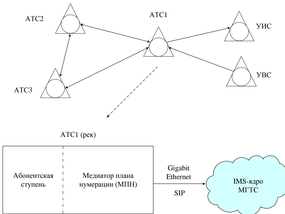
Рис. 1. Структура координатной АТС после ее модернизации
