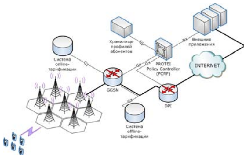
Рис. 1. PROTEI Policy Controller в сети 3GPP Release 7
